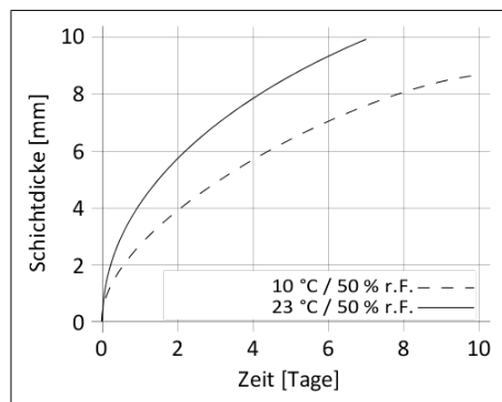
Diagramm 1: Durchhärtengeschwindigkeit Sikaflex®-508
