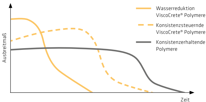
Konsistenzkurven ausgewählter PCEs
