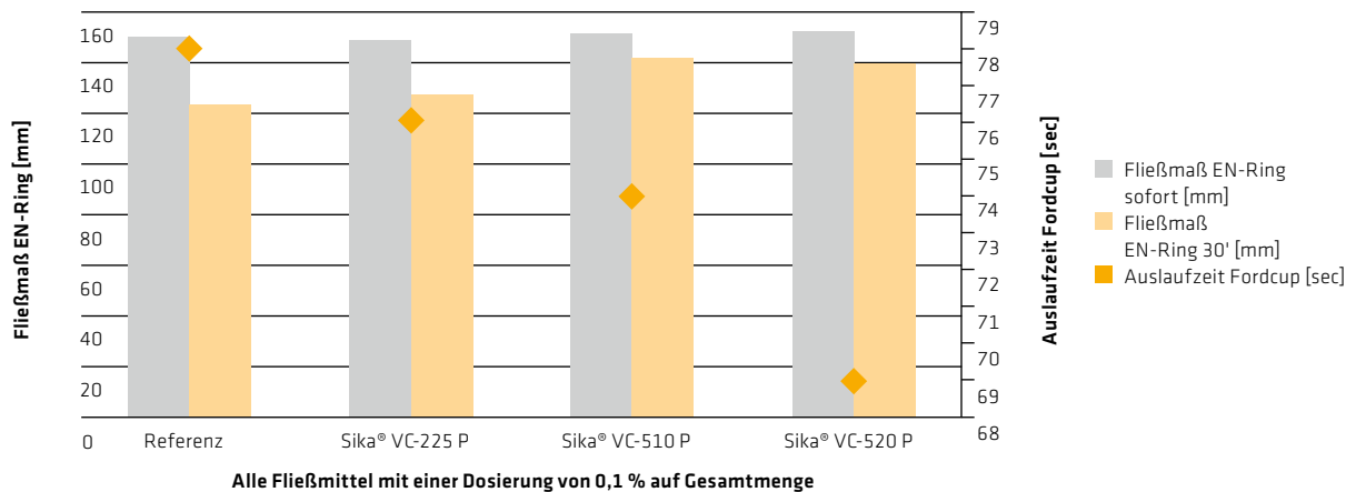
Fließmaß über die Zeit und Viskosität der Mischung
