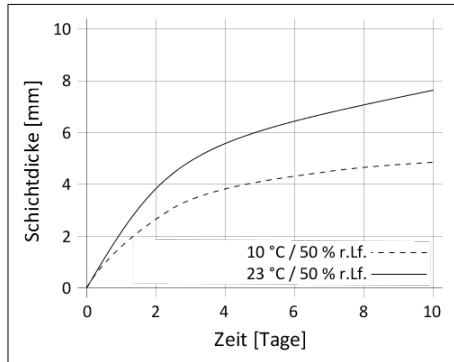
Diagramm 1: Durchhärtengeschwindigkeit Sikaflex®-529 Evolution
