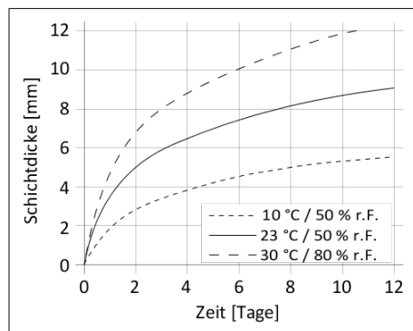
Diagramm 1: Durchhärtgeschwindigkeit von Sikaflex®-260 N
