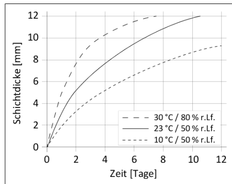
Diagramm 1: Durchhärtengeschwindigkeit Sikaflex®-821 FR
