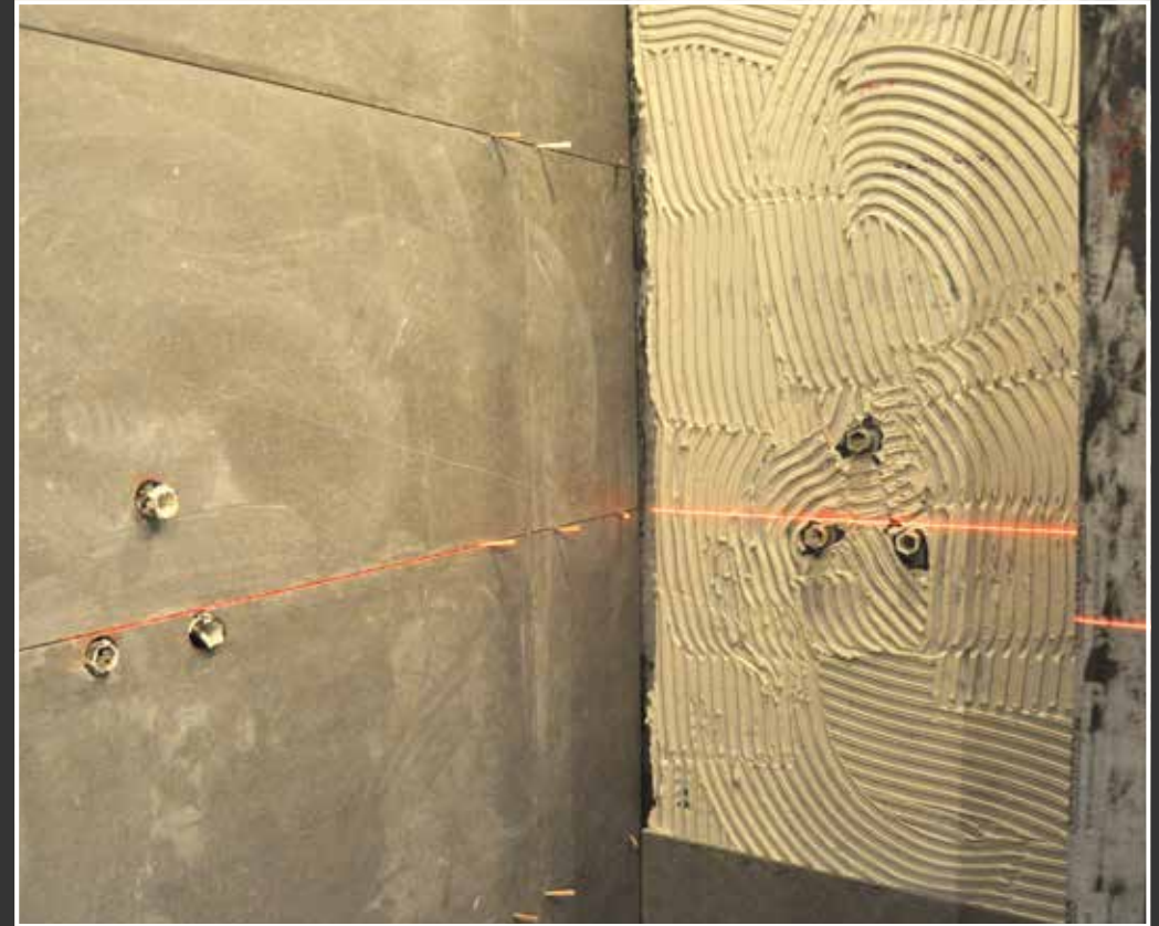
Auf der AIV-B kam SCHÖNOX Q6W zur Anwendung.
