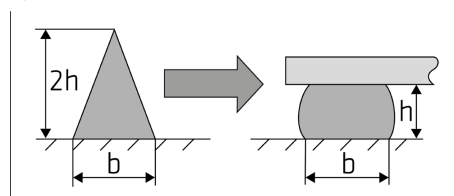
Abbildung 1: Empfohlener Klebstoffauftrag
