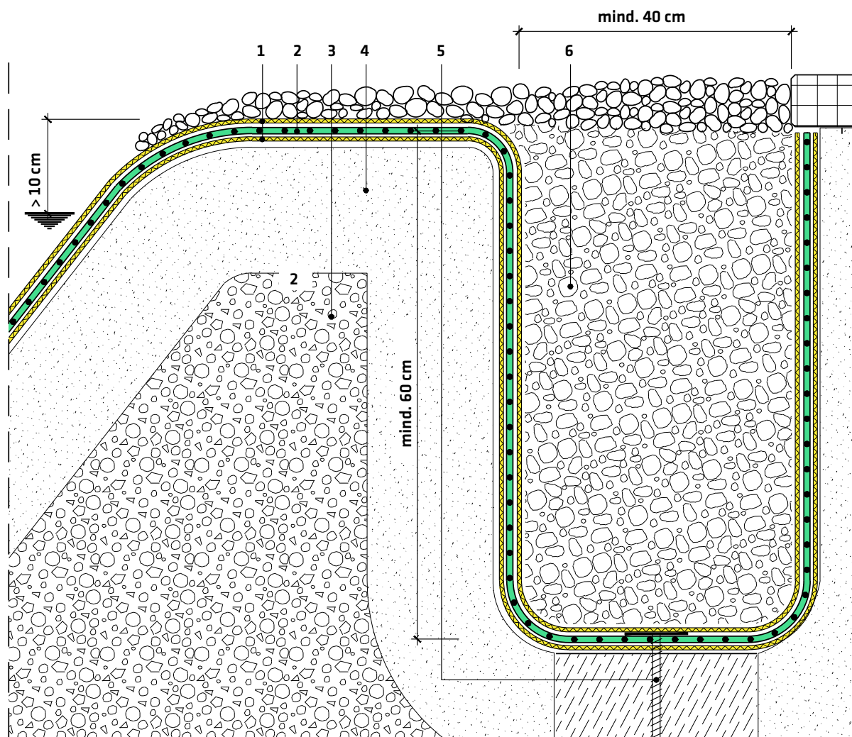
Detail 1.5 | Randabschluss mit Einbindegraben
