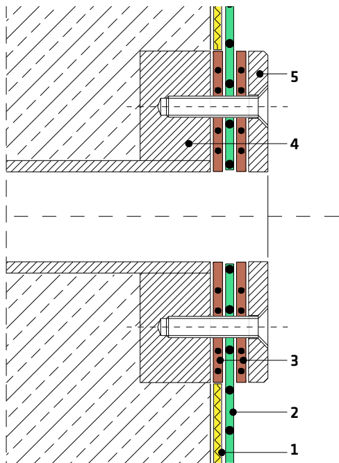
Detail 3.1 | Einströmdüse (Los- und Festflanschverbindung)
