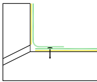
Detail 4.5 Seite 51
