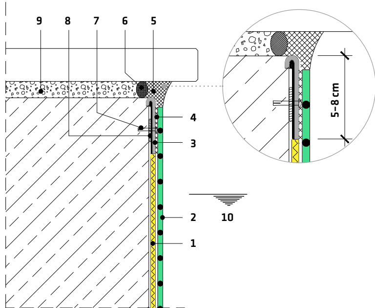
Detail 1.1 | Randabschluss auf vertikales Sikaplan
