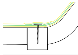
Detail 4.6 Seite 52
