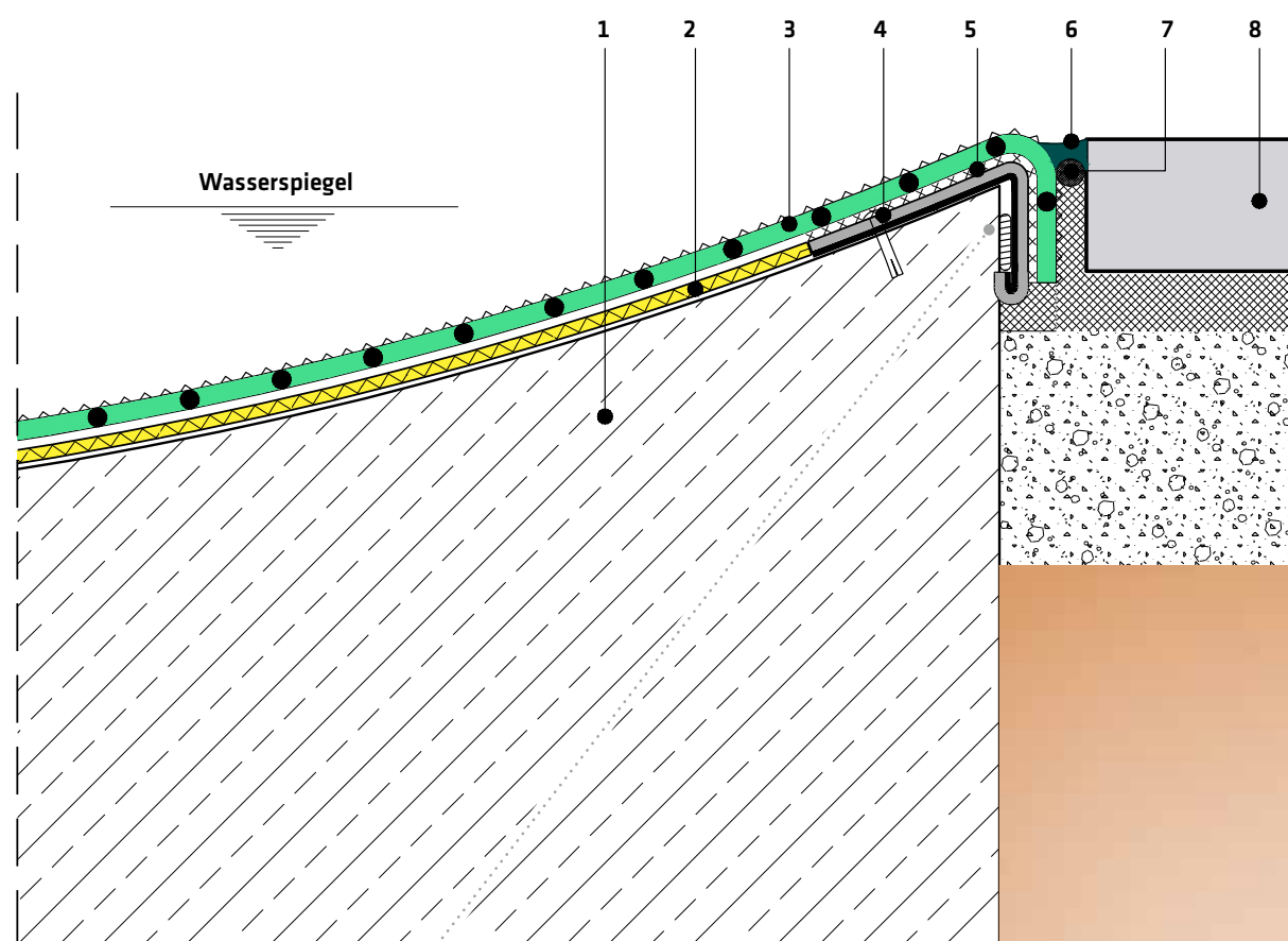
Detail 1.7 | Randabschluss Kinderbecken
