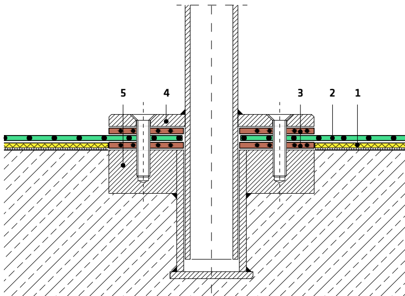
Detail 3.3 | Los-/Festflanschverbindung
