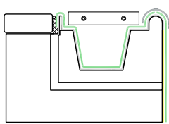
Detail 1.6 Seite 39
