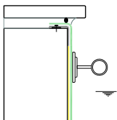
Detail 1.6 Seite 39
