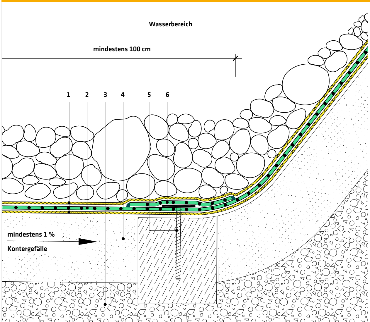
Detail 4.6 | Kehlbereich
