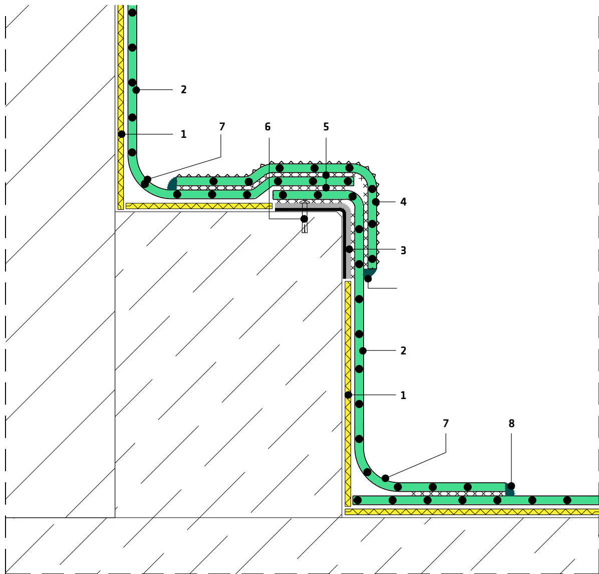
Detail 2.2 | Stehstufe
