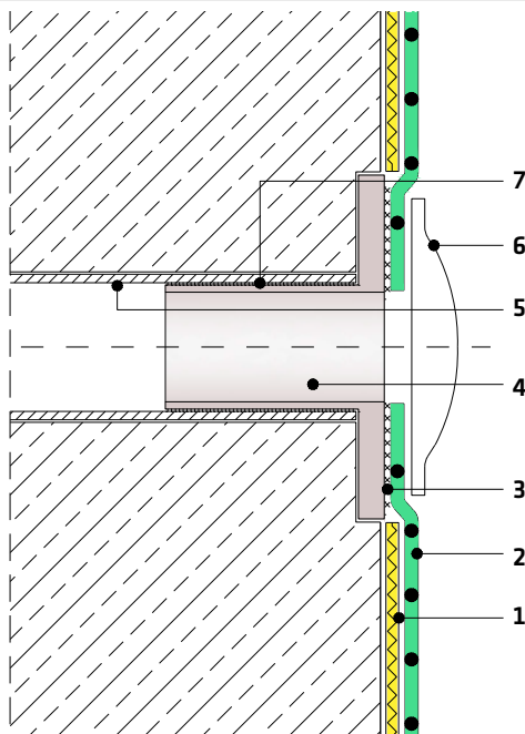
Detail 3.2 | Aufschweißflansch
