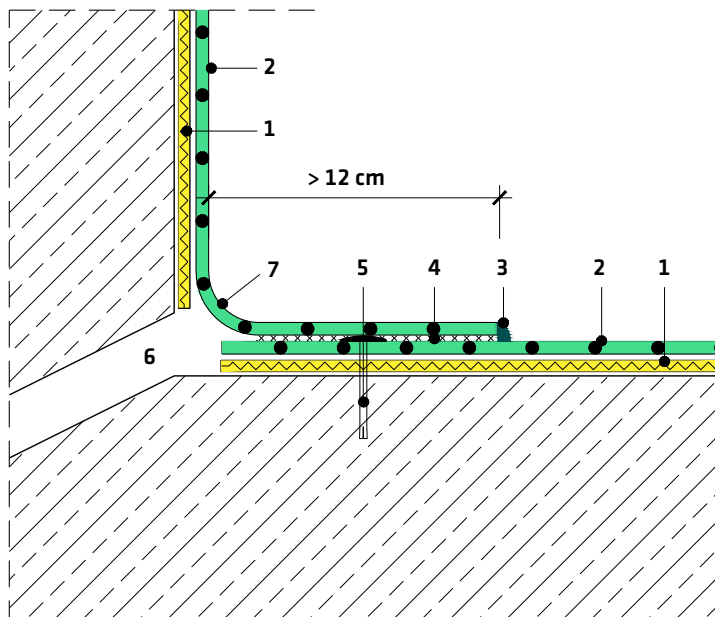
Detail 4.1 | Übergang Wand-Boden
