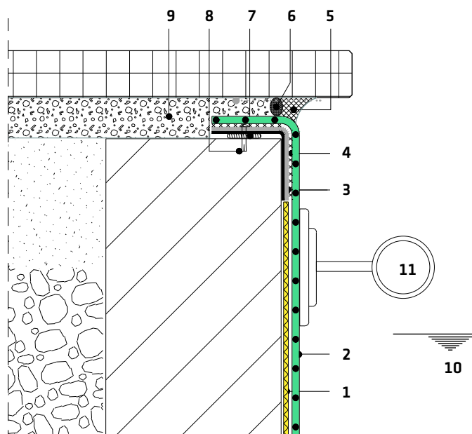
Detail 1.2 | Randabschluss auf Sikaplan® WP/WT Verbundblechwinkel
