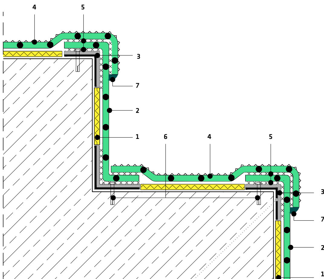
Detail 2.1 | Treppenstufe - erweitertes Verlegesystem
