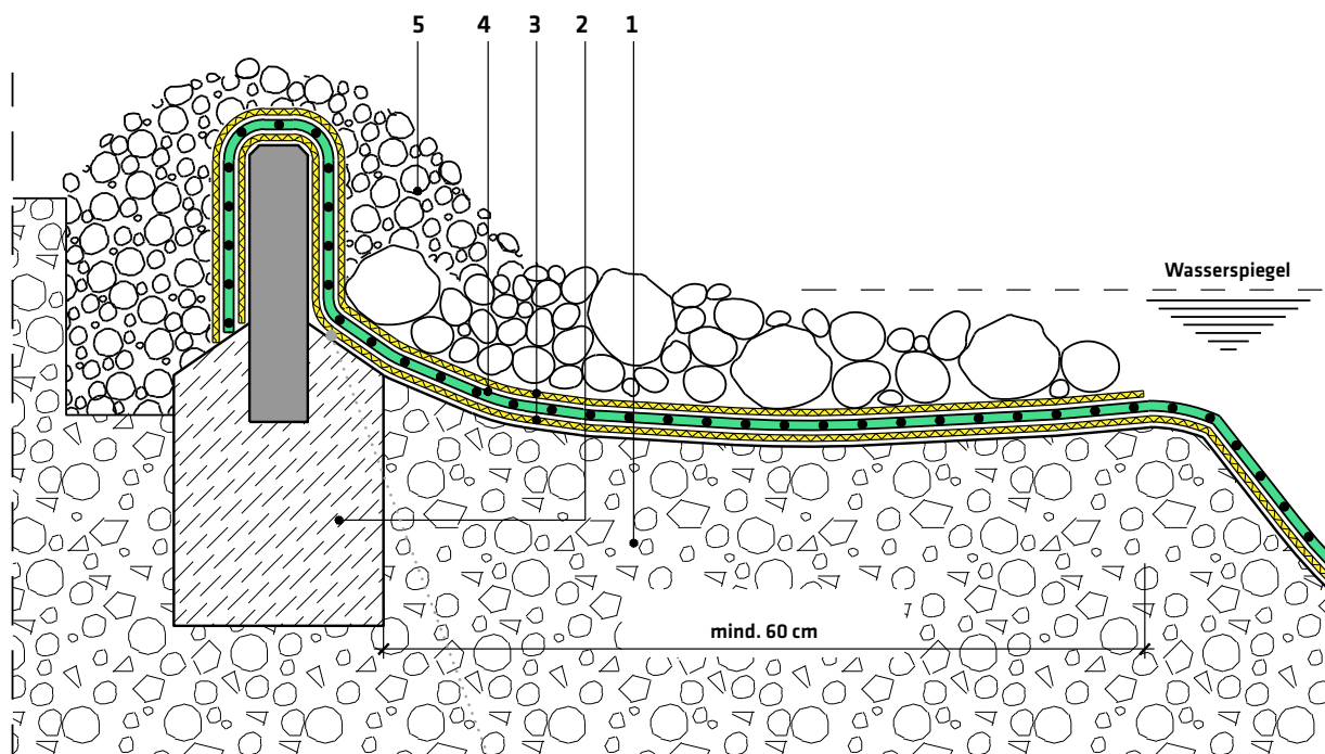
Detail 1.9 | Teichrandabschluss mit Randstein
