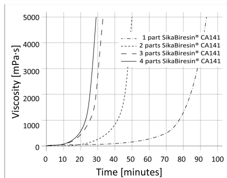
Diagramm 1: Viskositätsentwicklung bei 80 °C in Abhängigkeit von der Beschleunigermenge
