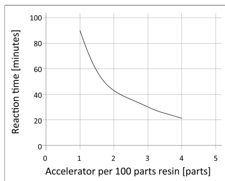
Diagramm 2: Reaktionszeit bei 80 °C in Abhängigkeit von der Beschleunigermenge, Gelnorm (CQP021-5 / IOS 9396)
