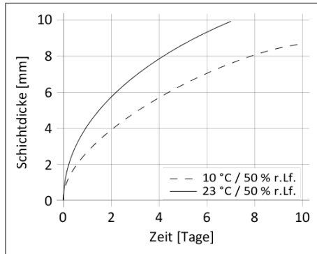
Diagramm 1: Durchhärtageschwindigkeit SikaTack®-MOVE Transportation
