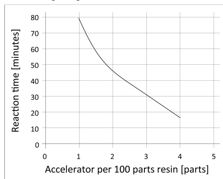
Diagramm 2: Reaktionszeit bei 100 °C in Abhängigkeit von der Beschleunigermenge, Gelnorm (CQP021-5 / IOS 9396)
