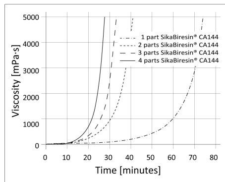
Diagramm 1: Viskositätsentwicklung bei 100 °C in Abhängigkeit von der Beschleunigermenge
