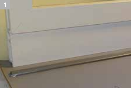
1 Anschluss der Flächenabdichtung (z. B. Sarnafil FPO PP) am Fensterelement Hart PVC.
