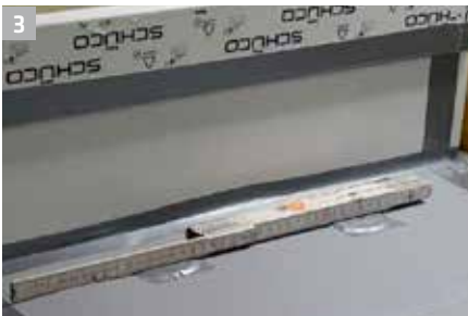
3 Abzuidichtenden Bereich mit Klebeband abgrenzen, Tellerbefestiger mit Klebeband PE Oberfläche entkoppeln.
