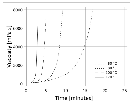
Diagramm 1: Viskositätsentwicklung
