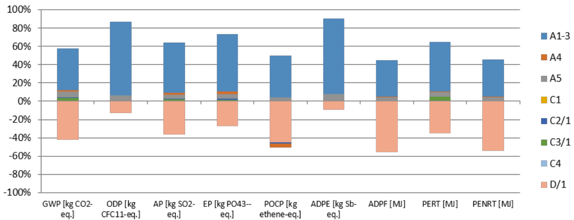
Relative Beiträge der Module zu den Umweltwirkungen und Primärenergieeinsatz von 1 m 2 Sarnafil® TS 77-20 E (100 % stoffliches Recycling)
