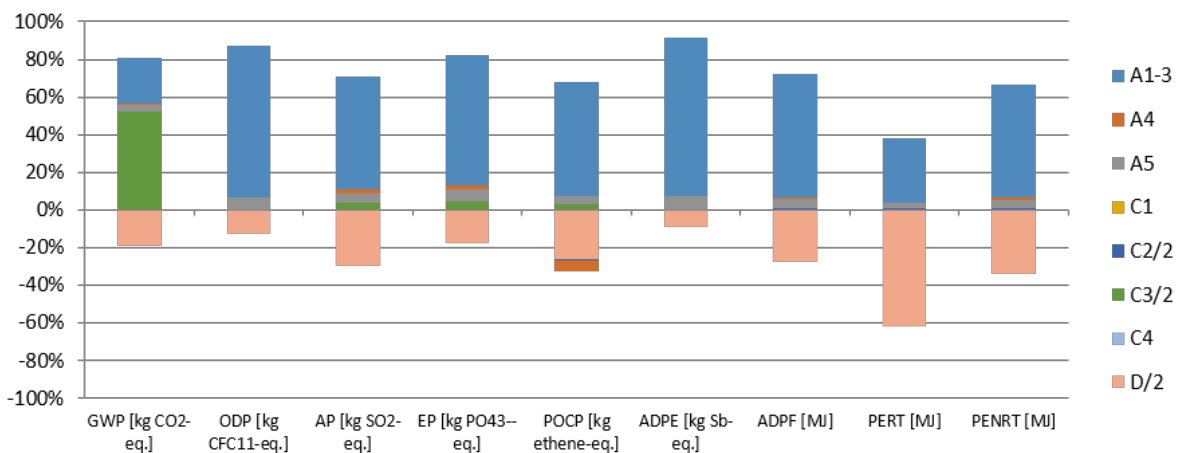
Relative Beiträge der Module zu den Umweltwirkungen und Primärenergieeinsatz von 1 m 2 Sarnafil® TS 77-20 E (100 % thermische Verwertung)
