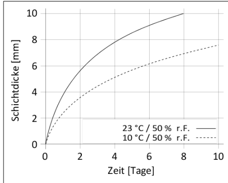
Diagramm 1: Durchhärtengeschwindigkeit von Sikaflex®-291i
