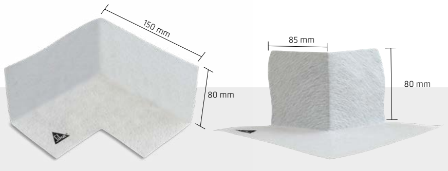
Vliesinnenecke
